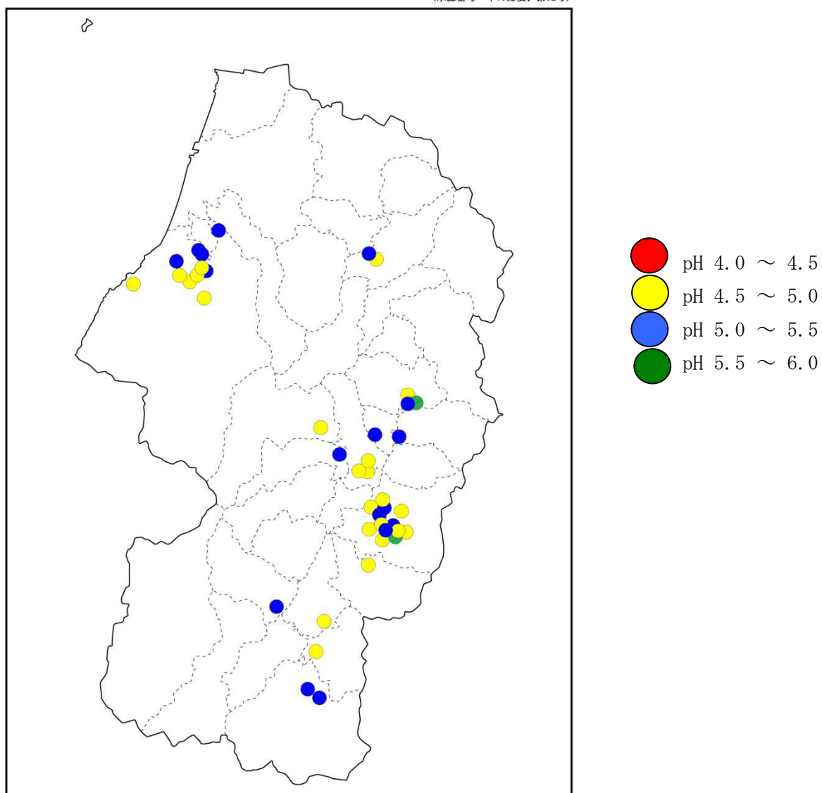
-1 pH の分布
