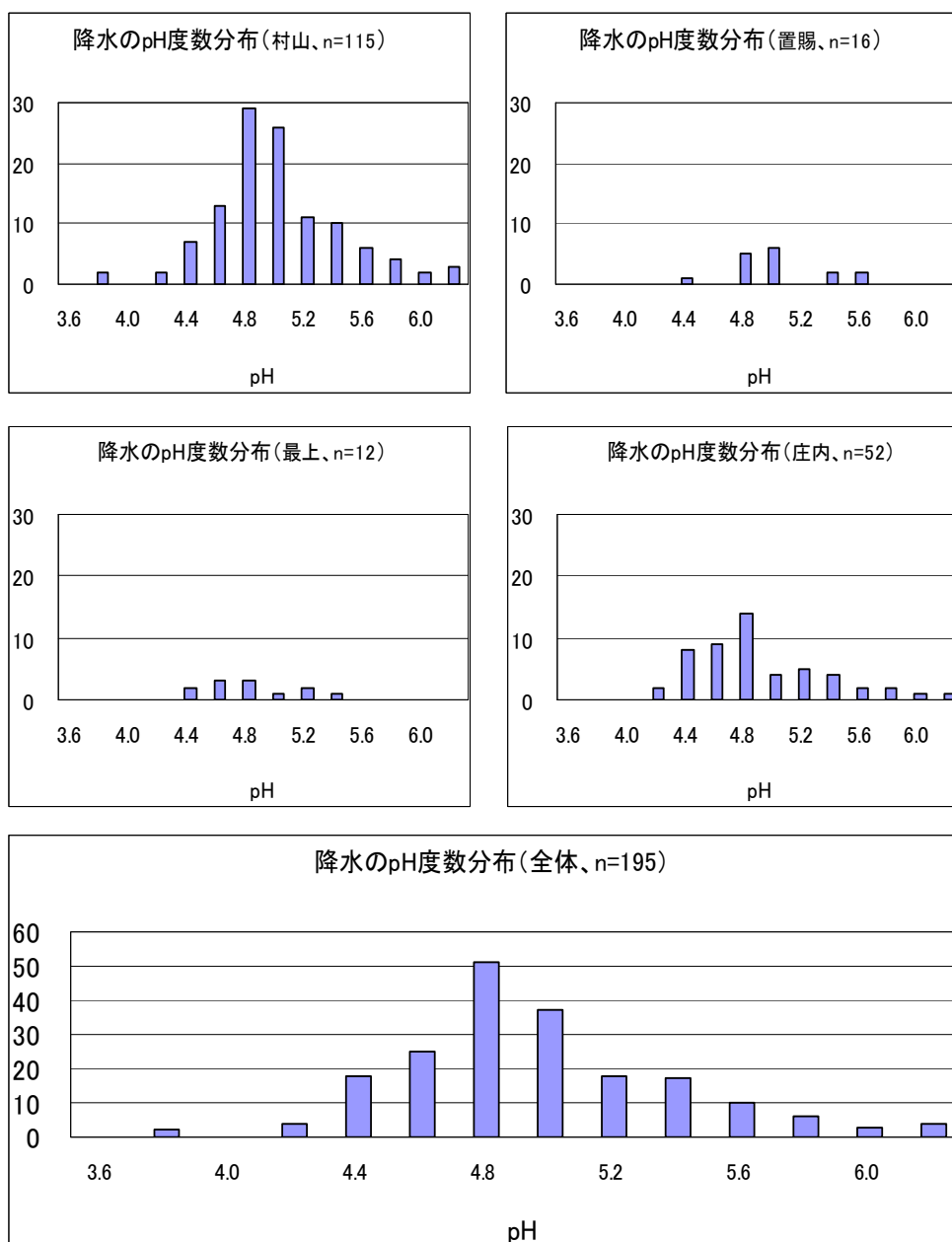
図-2 降水の pH の度数分布
