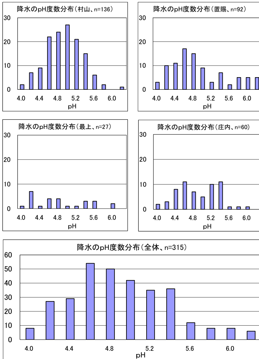
図-2 降水の pH の度数分布
