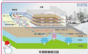
帯水層蓄熱冷暖房システム模式図
