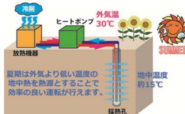
地中熱HP冷暖房
