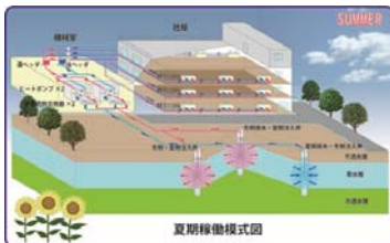
帯水層蓄熱冷暖房システム
