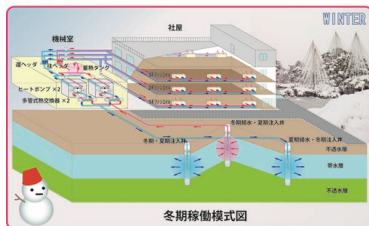
帯水層蓄熱冷暖房システム模式図
