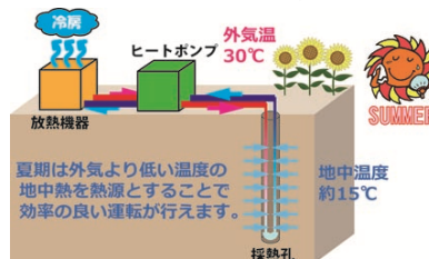
地中熱HP冷暖房
